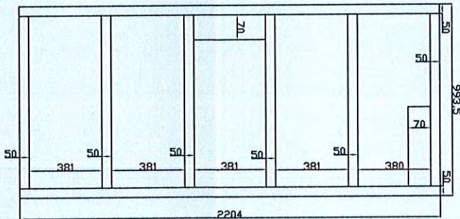
门框示意图
